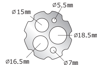
<集塵パッド用プレート38A> 品番：SJP038PA
