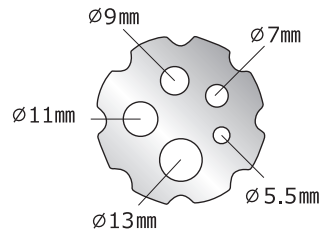
<集塵パッド用プレート38> 品番：SJP038P
